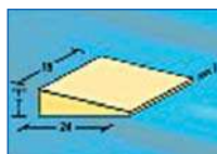
Ék alakú, 20°, 24x18x7/1 cm(81512)
