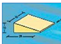
Ék alakú, 20°, 28x18x10/1 cm (81532)
